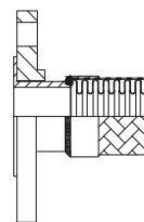
Swivel flange "D" Flangia girevole "D"
