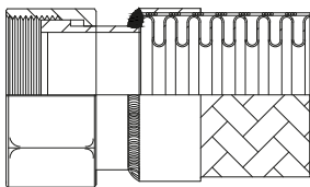
Swivel female flat seat Femmina girevole sede piana
