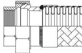
Union Coupling Bocchettone a tre pezzi
