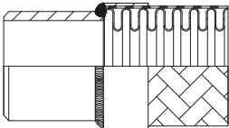
Welding end Manicotto liscio a saldare
