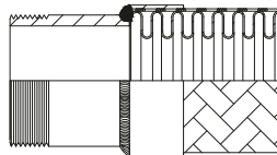
Threaded male end Tronchetto filettato
