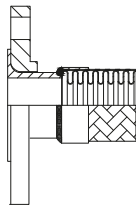
Swivel flange "C" Flangia girevole "C"
