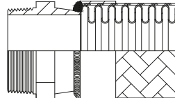
Fixed male Maschio fisso
