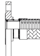
Flangia fissa "A" Fixed flange "A"
