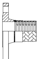
Flangia fissa "B" Fixed flange "B"
