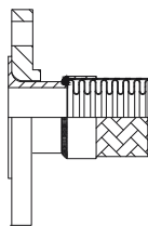
Flangia girevole "C" Swivel flange "C"
