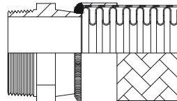
Maschio fisso Fixed male
