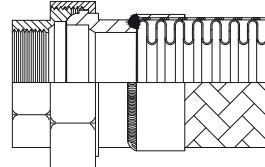
Bocchettone a tre pezzi Union Coupling
