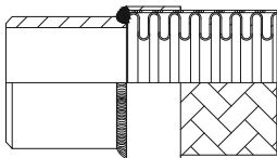
Manicotto liscio a saldare Welding end
