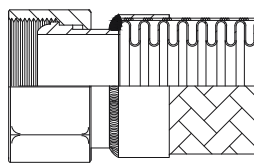
Femmina girevole sede ogiva Swivel female cone seat
